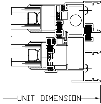
14 DH SERIES @ JAMB
